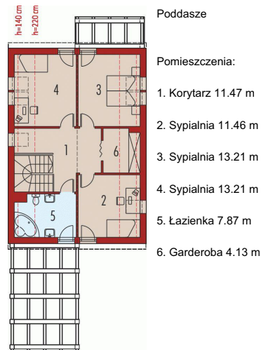
Poddasze
