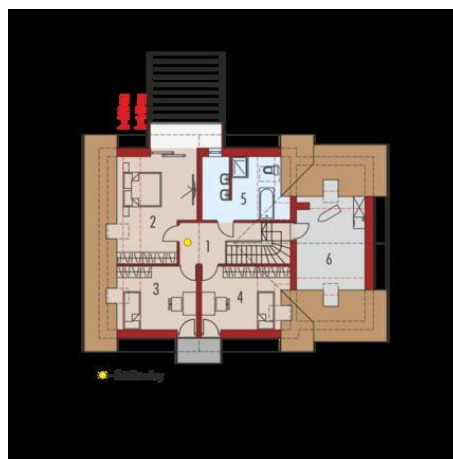
Poddasze
