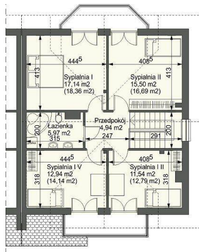
Poddasze
