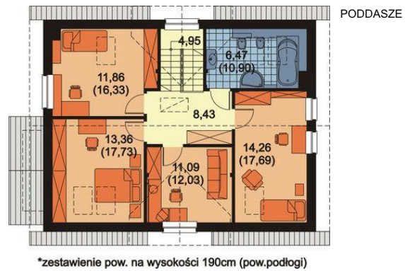
Poddasze
