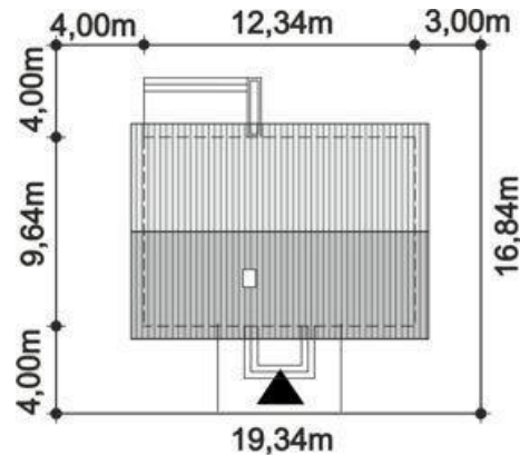
RZUT PARTERU: pow. pomieszczeń 83,89m 2
