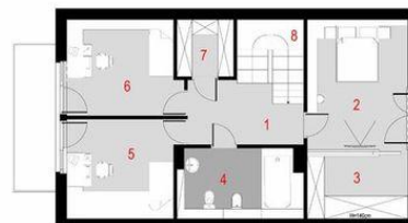
Poddasze
