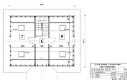
Poddasze
