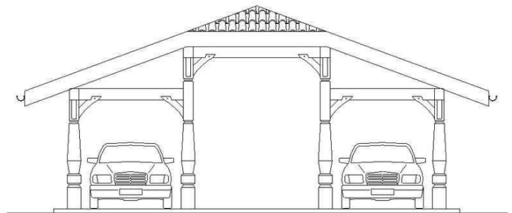
ELEWACJA FRONTOWA
