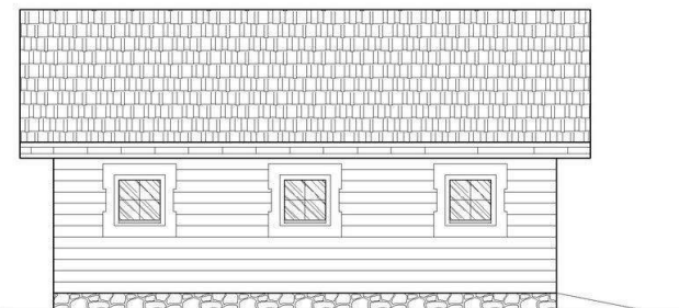
ELEWACJA BOCZNA
