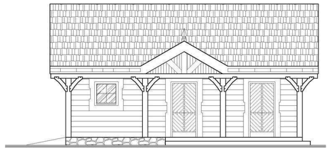
ELEWACJA BOCZNA
