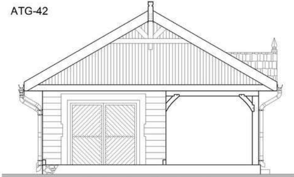
ELEWACJA FRONTOWA
