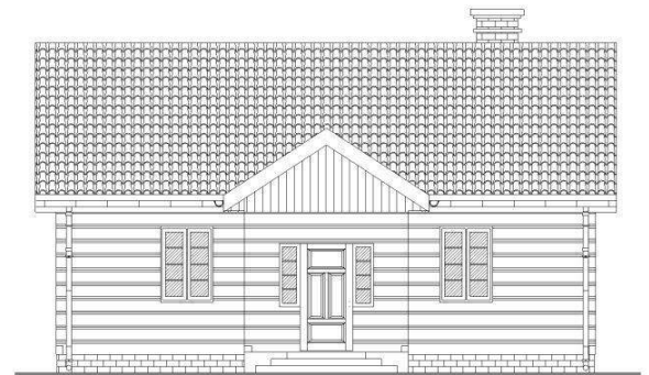
ELEWACJA FRONTOWA
