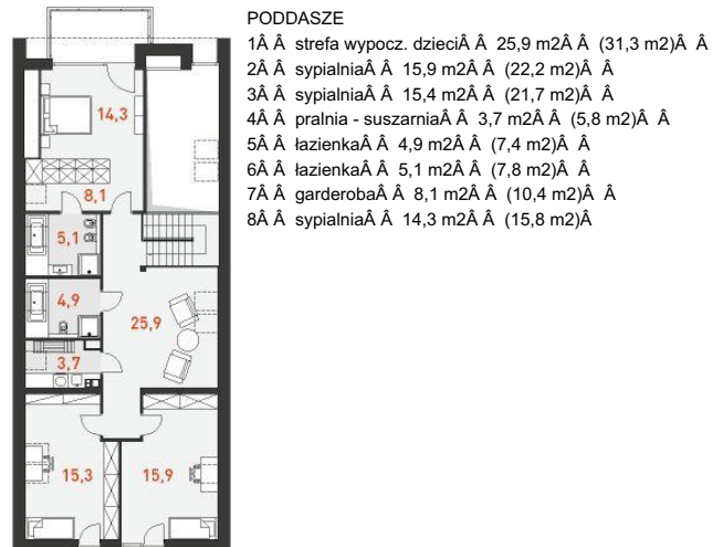
Poddasze
