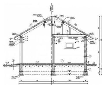
Przekrój A-A
