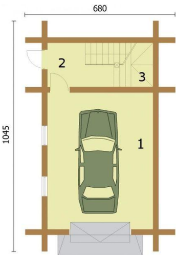
Rzut przyziemia 1. Garaż 29.76m 2 2. Komunikacja 7.16m 2 3. Schowek 1.8m 2
