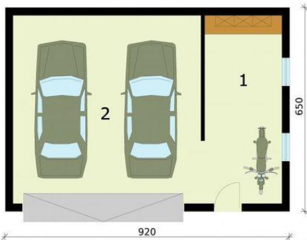
Rzut przyziemia 1. Pom. gospodarcze 15m 2 2. Garaż 36.48m 2
