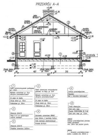
Przekrój A-A
