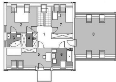
Poddasze
